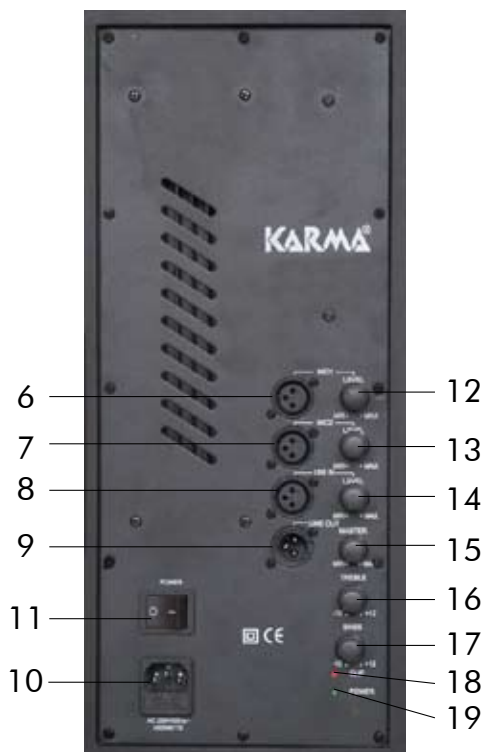
Pannello BX 6012A e BX 6015A
