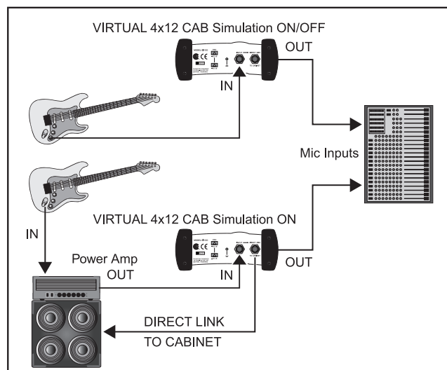
Fig. 2.1: 1. Chitarra → box DI → banco di mixaggio 2. Chitarra → amplificatore a valvole → box DI → cassa altoparlanti/banco di mixaggio
