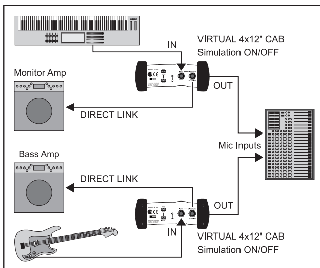
Fig. 2.2: 1. Chitarra basso → box DI → amplificatore/banco di mixaggio 2. Tastiera → box DI → amplificatore/banco di mixaggio
