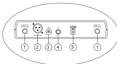
BASE RICEVENTE (SET 7510 e SET 7510LAV)
