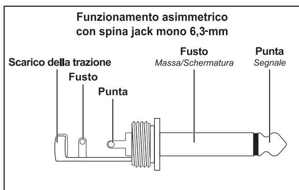
Fig. 2.3 Connettore jack TS da ¼"
