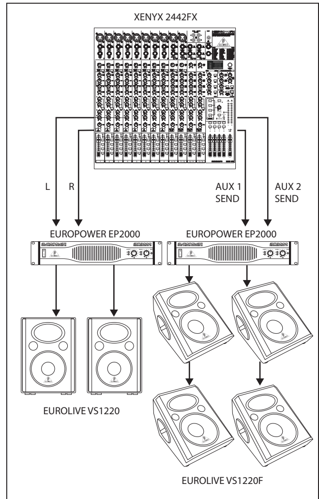
Fig. 5.2 Sistema stereo Full-range con floor-monitor
