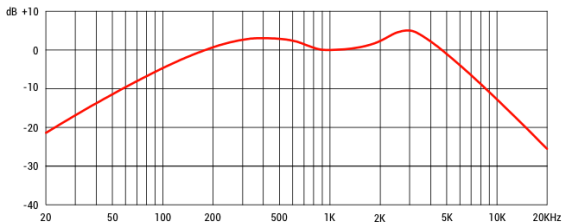
频率响应曲线
